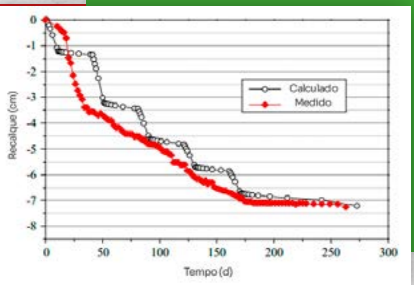
Figura 8 - Valores calculados e medidos do processo de recalque.
