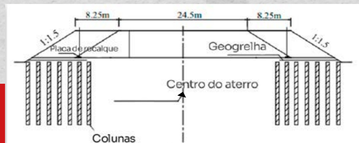
Fig 7 - Localização das placas de recalque.
