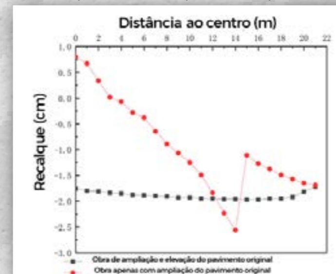
Figura 4- Diagrama do recalque total do aterro ao final da obra
