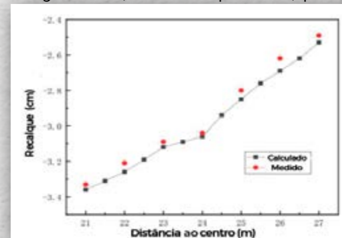
Figura 6 - Valores do recalque calculado e medido
